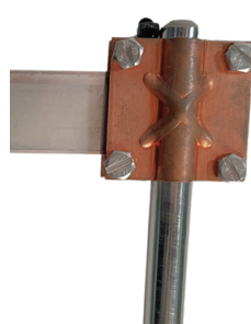
Réf. 16125 Collier de raccordement en cuivre Pour conducteurs plats
