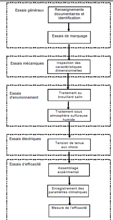
Figure C.1 – Déroulement des essais
